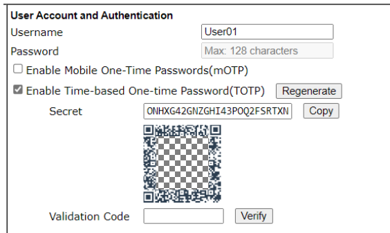
Ein Benutzerkonto auf dem VPN Gateway einrichten QR-Code und/oder Secret dem Benutzer geben
